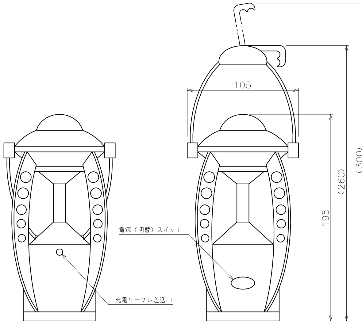
充電式LEDランタン
