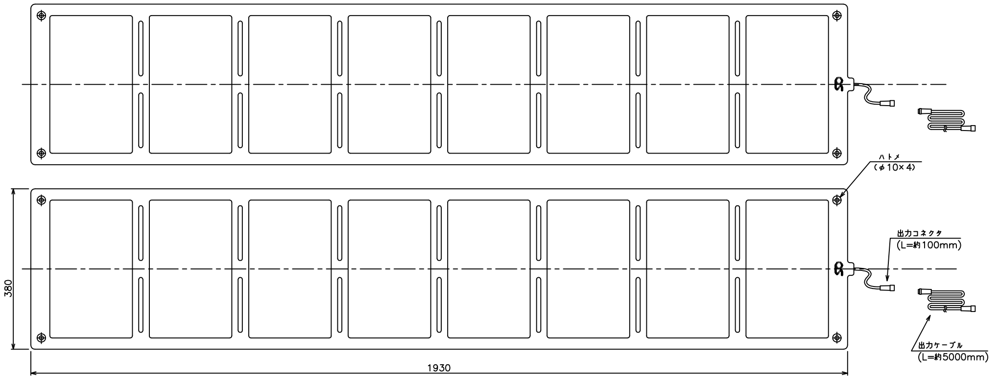
ソーラーシート 380×1930×3 (突起部は除く)
