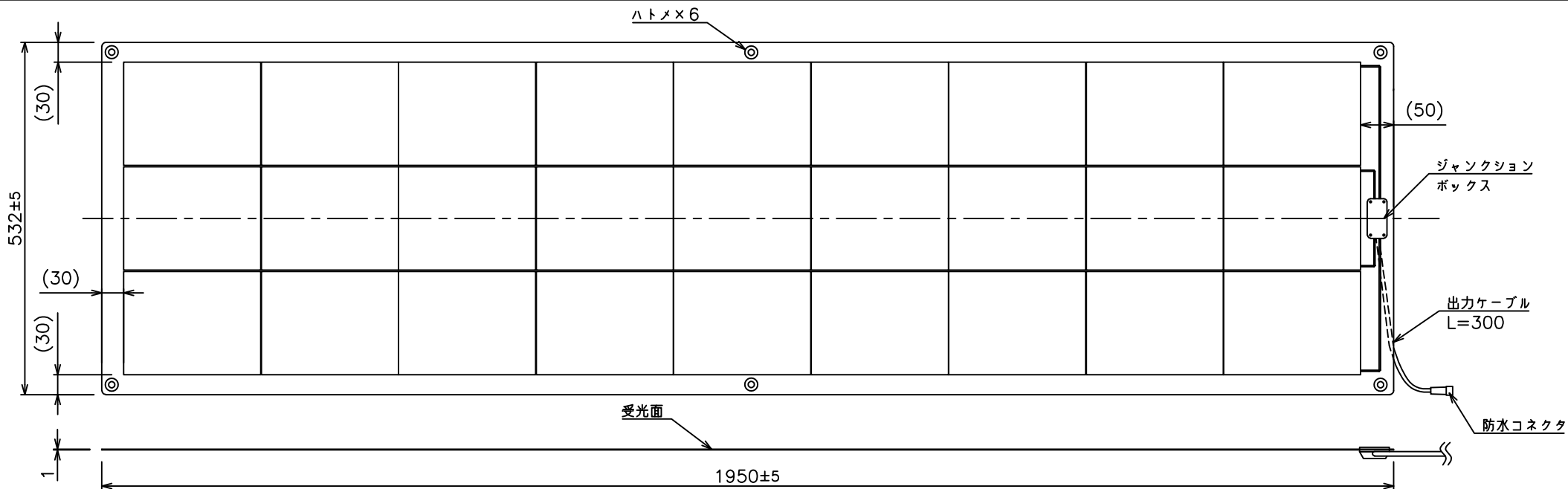
モバイルソーラーシート
