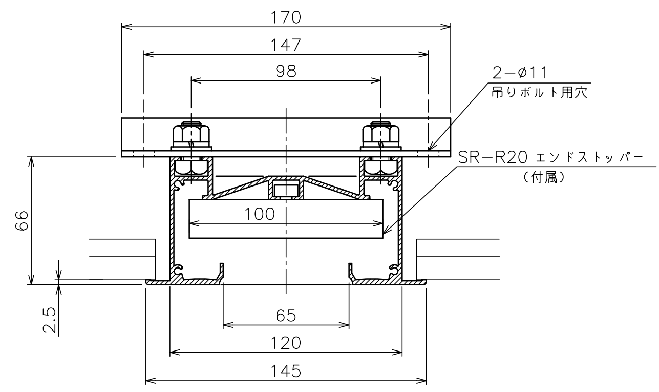
”c”部詳細
