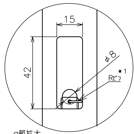
φ部拡大 脱落防止ワイヤー、Rピン差し込み穴 *1 固定ボルト脱落防止用
