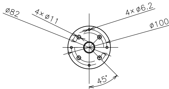
天井取付穴寸法
