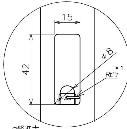
○部拡大 脱落防止ワイヤー、Rピン差し込み穴 *1 固定ボルト脱落防止用
