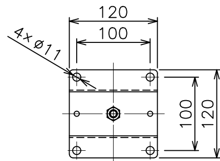
天井取付穴寸法
