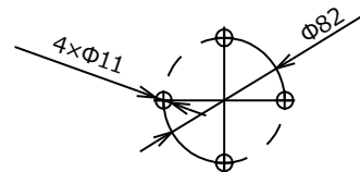
取り付け用孔寸法
