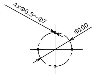
取り付け用孔寸法
