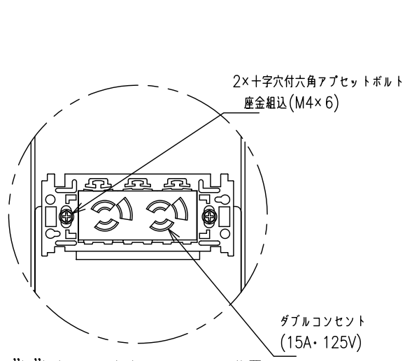
"b"矢視図 (ダブルコンセント位置) ダブルコンセントはボックスカバーを取り外したボックス本体内部にあります。
