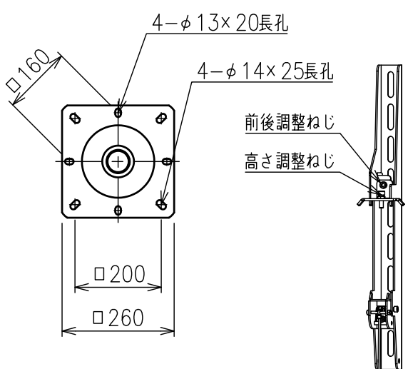
矢視 A - A スラブ取付板 (オプション)
