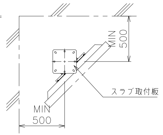
取付位置参考図 (ディスプレイW949の場合)
