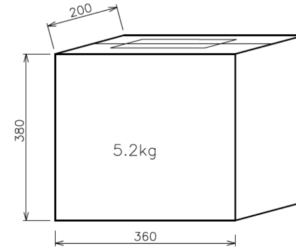
梱包仕様図(1/8)
