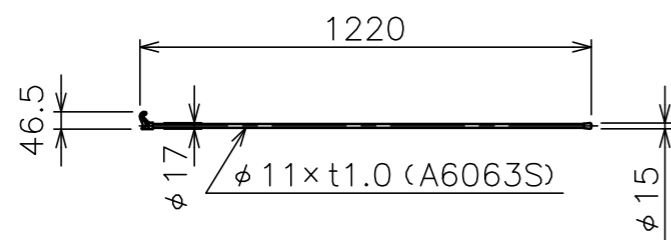
フック棒HK-1200A 質量0.11kg
