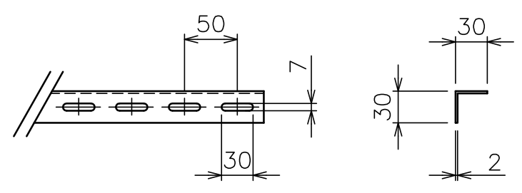
スクリーン取付金具詳細
