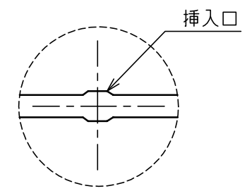
b部 M10ボルト挿入口拡大図
