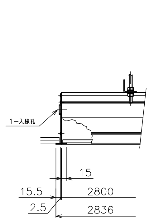
”a”部詳細
