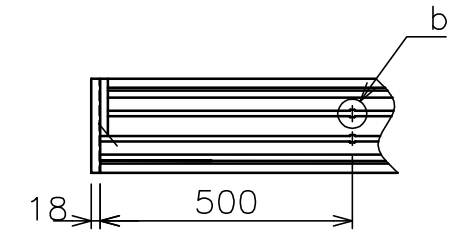
矢視 B
