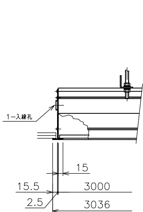
”a”部詳細
