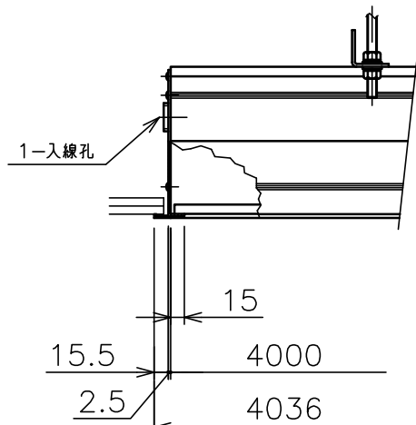
”a”部詳細
