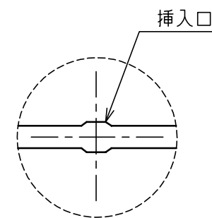
b部 M10ボルト挿入口拡大図
