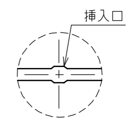
b部 M10ボルト挿入口拡大図
