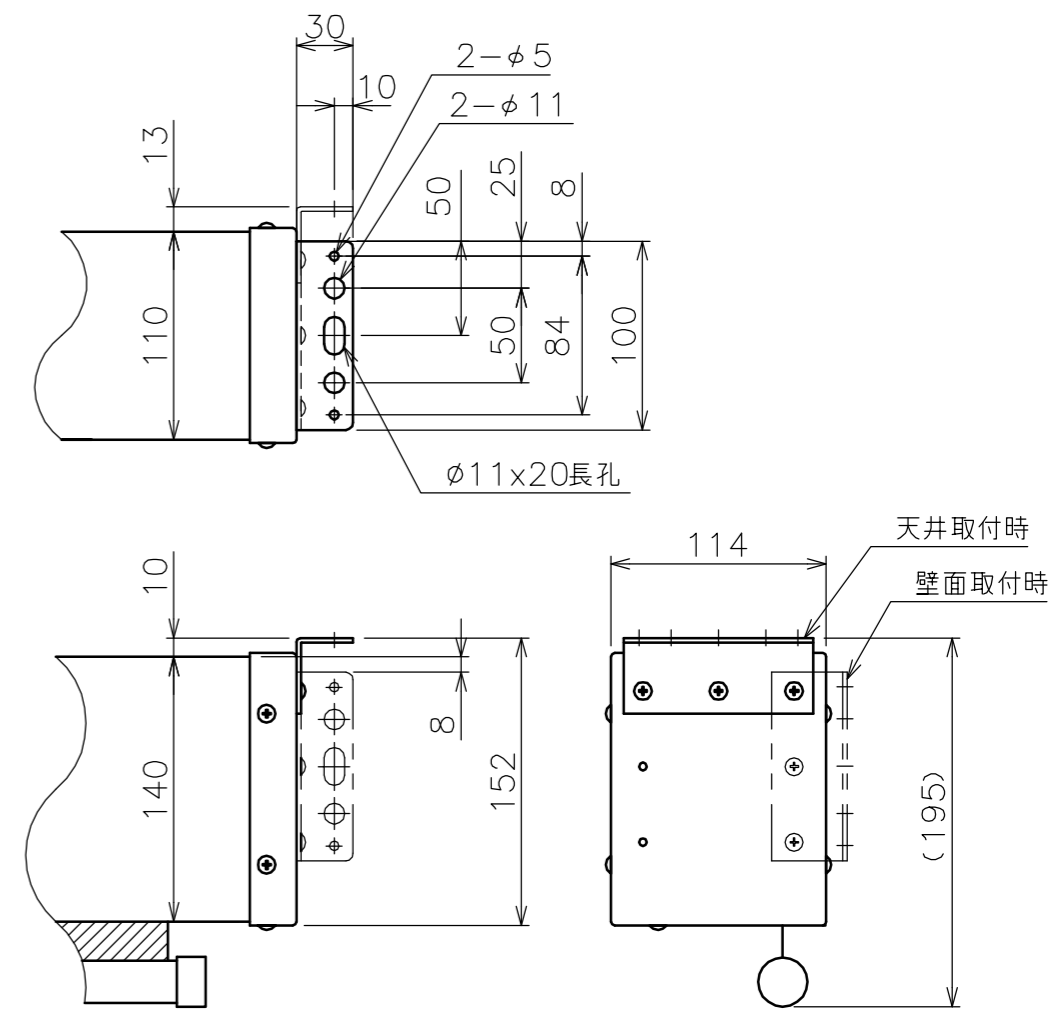
”a”部詳細
