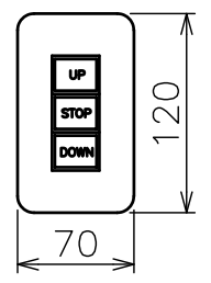
一連用埋込型スイッチ (モダンプレート: ミルキーホワイト)
