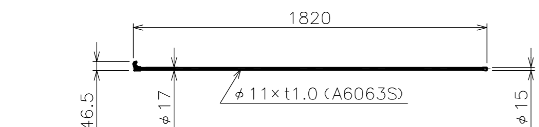
フック棒 HK-1800A 質量 0.16kg
