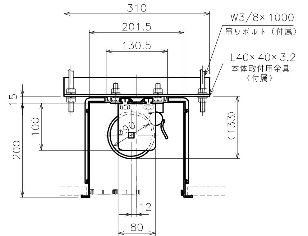
矢視 A - A
