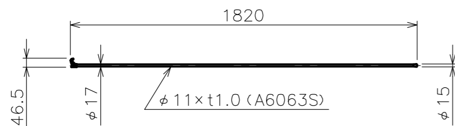
フック棒HK-1800A 質量0.16kg
