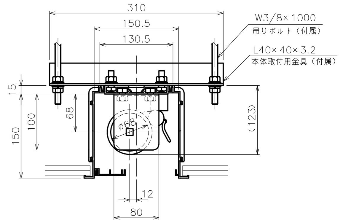
矢視 A - A
