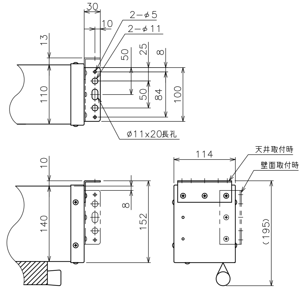
”a”部詳細
