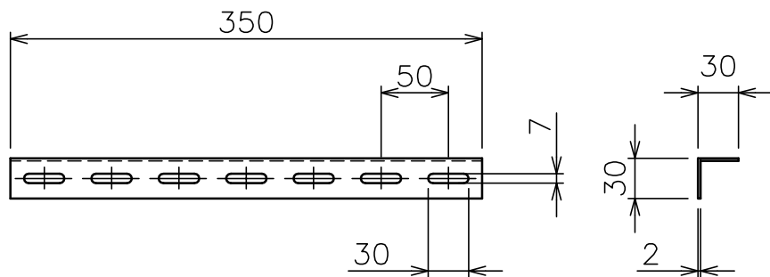
スクリーン取付金具詳細
