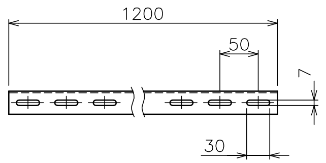
スクリーン取付金具詳細
