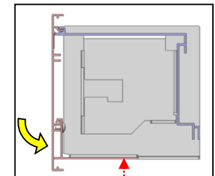
ねじ穴位置
