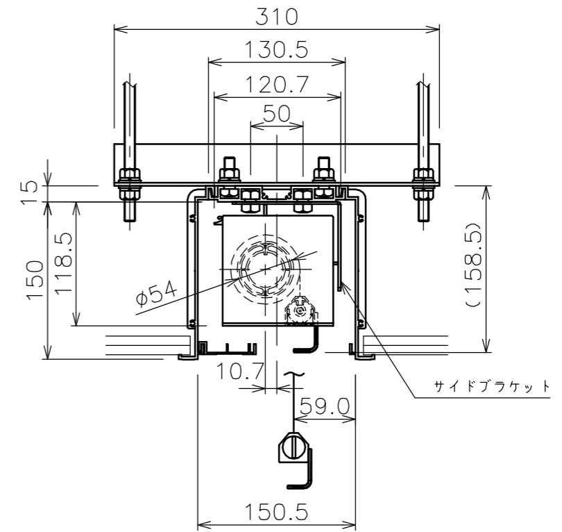
矢視A-A(S=1/5)
