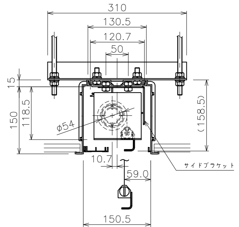
矢視A-A(S=1/5)
