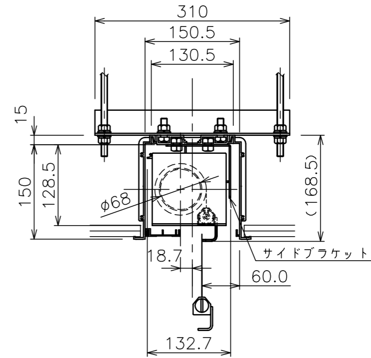
矢視A-A(S=1/6)
