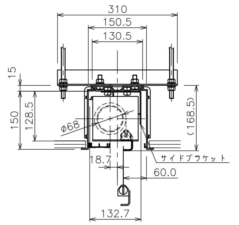
矢視A-A(S=1/6)
