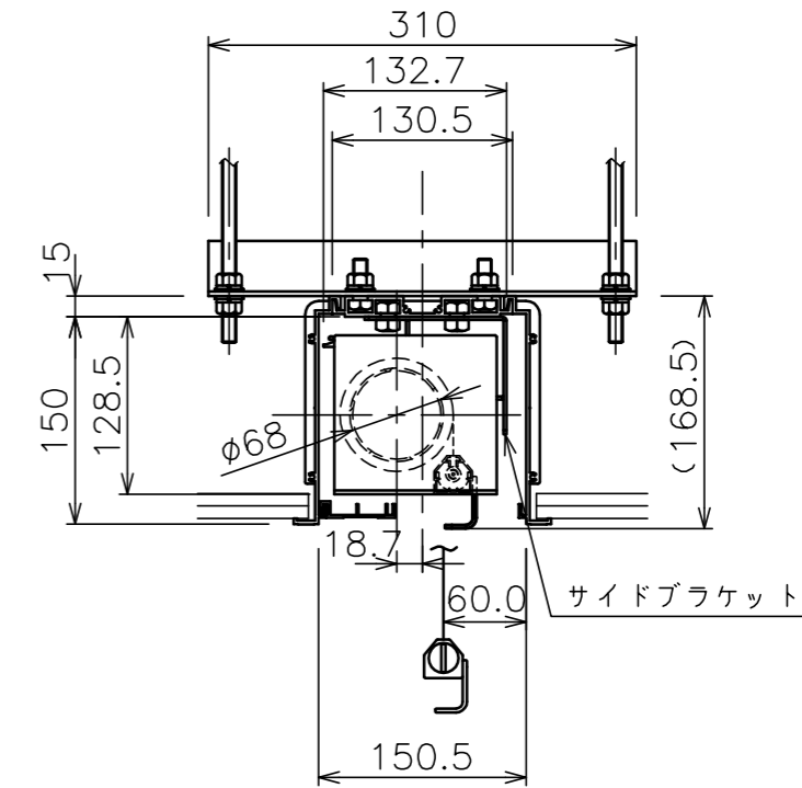
矢視A-A(S=1/6)
