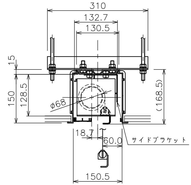
矢視A-A(S=1/6)
