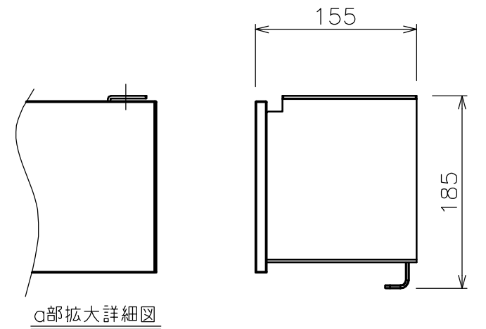
サイドブラケット(S=1/5)
