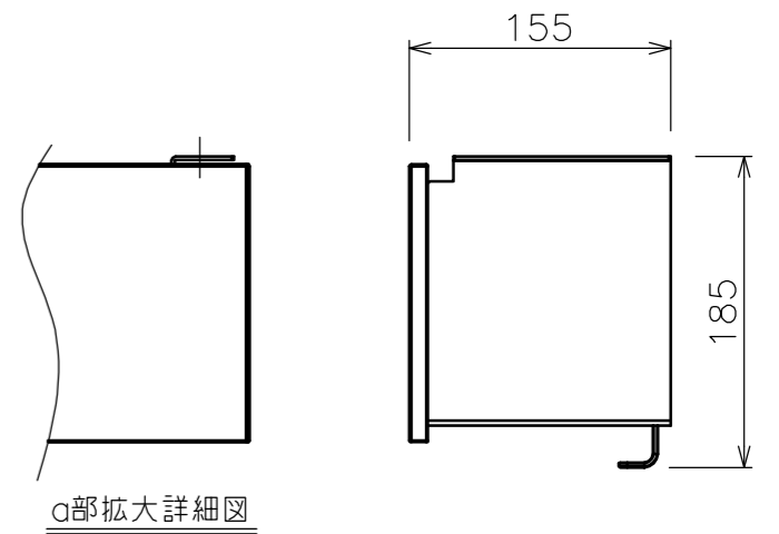
サイドブラケット(S=1/5)
