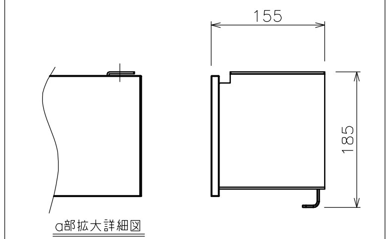
サイドブラケット(S=1/5)
