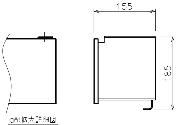
サイドブラケット(S=1/5)
