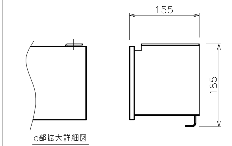
サイドブラケット (S=1/5)
