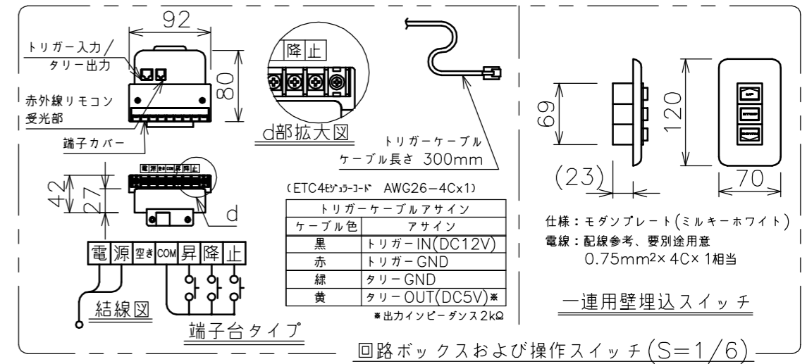
矢視A-A(S=1/6)
