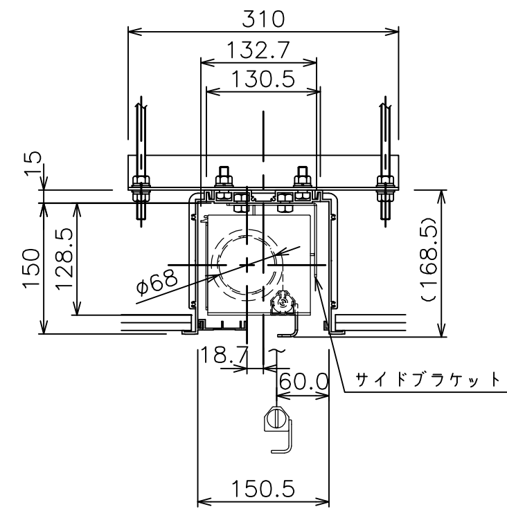
矢視A-A(S=1/6)
