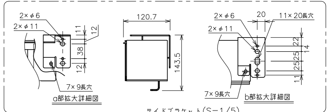
サイドブラケット (S=1/5)
