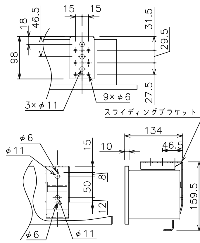
スライディングブラケット詳細図(S=1/5)
