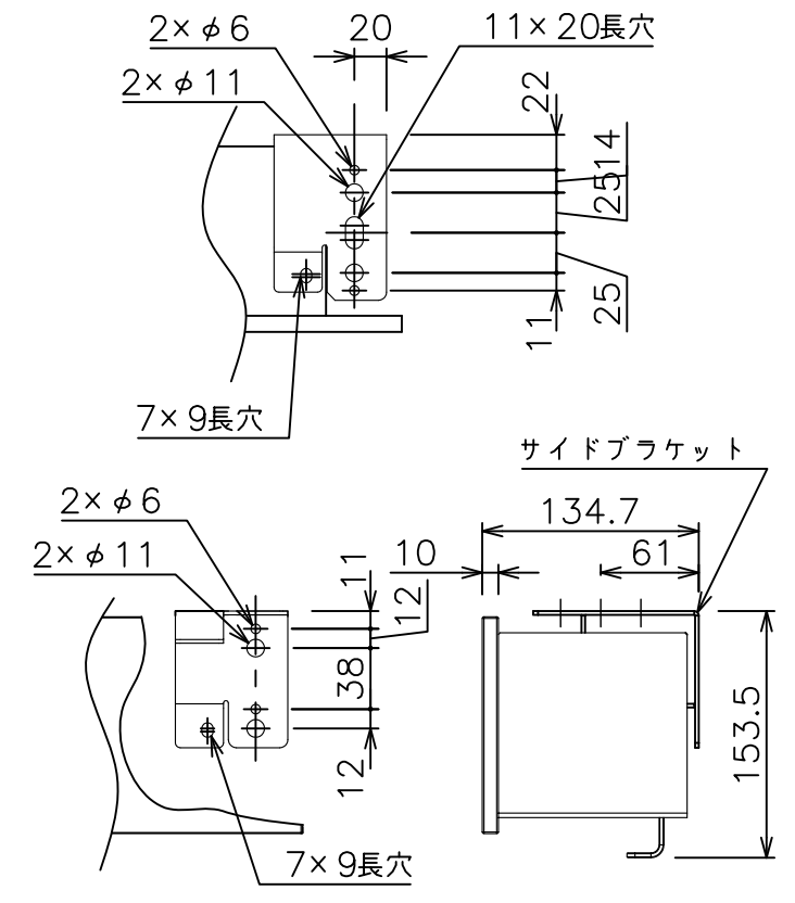
サイドブラケット詳細図(S=1/5)
