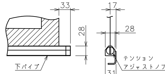
下パイプ詳細図(S=1/5)
