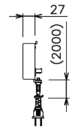
回路ボックスおよび操作スイッチ (S=1/6)
