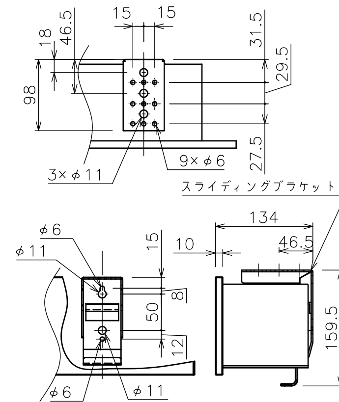
スライディングブラケット詳細図(S=1/5)
