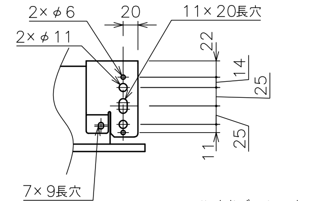
サイドブラケット
