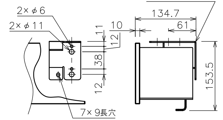
サイドブラケット
