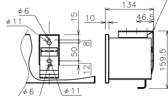
スライディングブラケット
