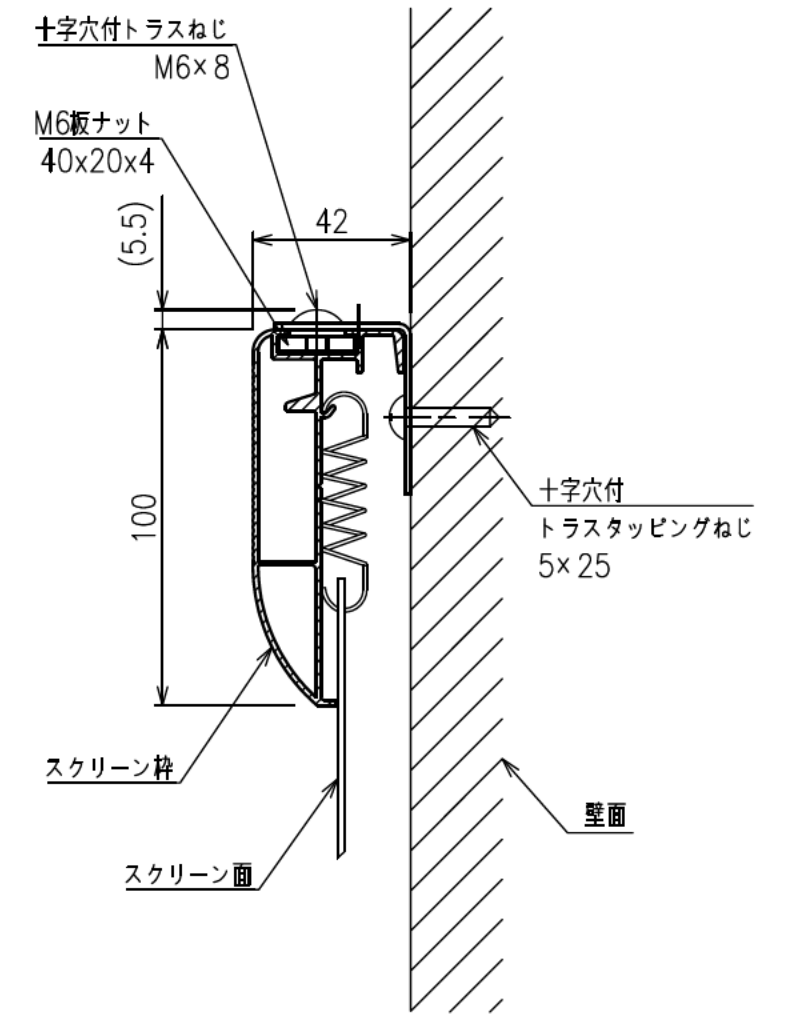
A-A断面拡大図
