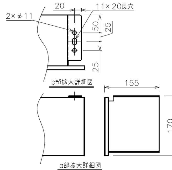
サイドブラケット(S=1/8)
