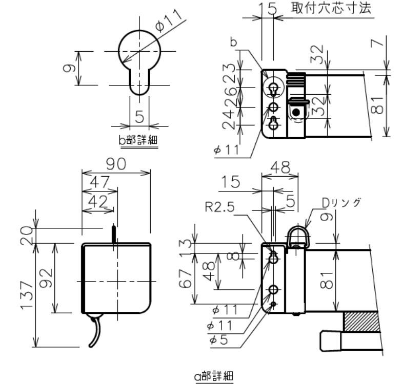
サイドキャップ詳細図 (S=1/5)
