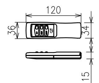
赤外線リモコン送信機/受光部
